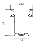
GU2716 - 27x16 mm Guida in alluminio
