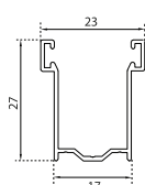
GU2817 - 2817x17 mm Guida in alluminio
