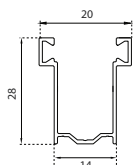
GU2814 - 28x14 mm Guida in alluminio
